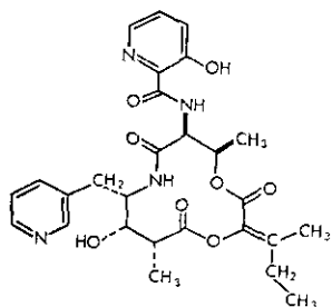
Pyridomycin (1970)
