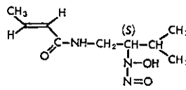
Dopastin (1973)
